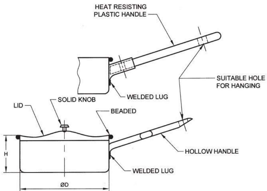
Fig. 9 Saucepan
